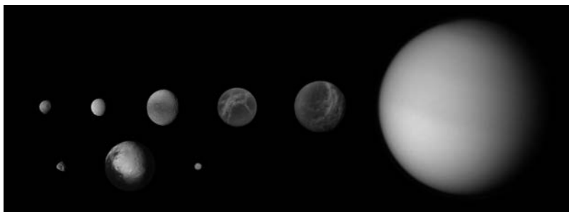
Рис. 1.4. Крупные спутники Сатурна.
