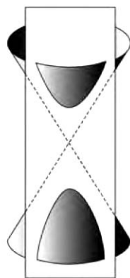
гипербола
