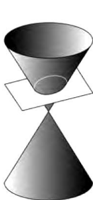
эллипс
