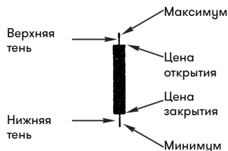
Рис. 2.4. Черное тело
