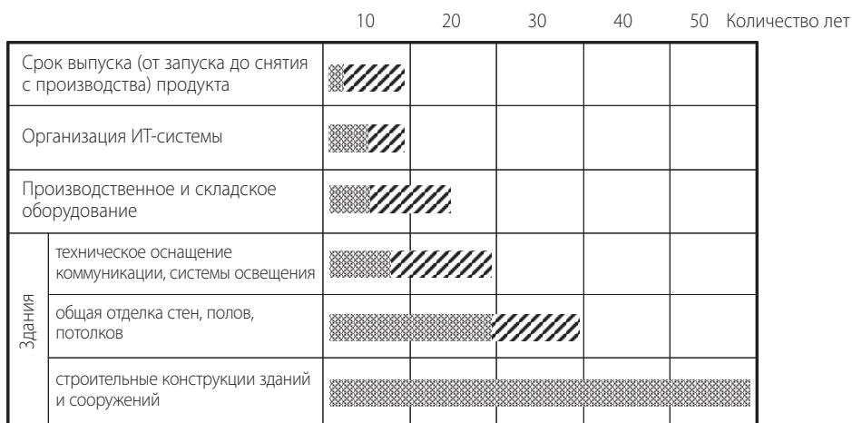
Рис. 2.4. Срок службы элементов завода
