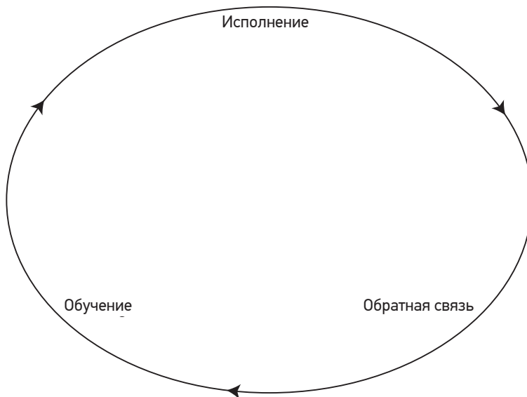
Рис. 1. Цикл обучения
